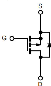
P-Channel MOSFET
