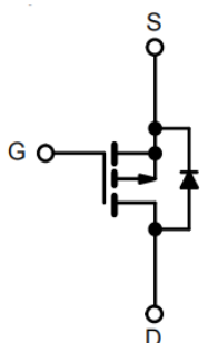
P-Channel MOSFET
