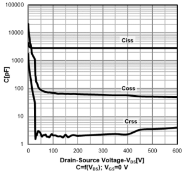
Typ. capacitances
